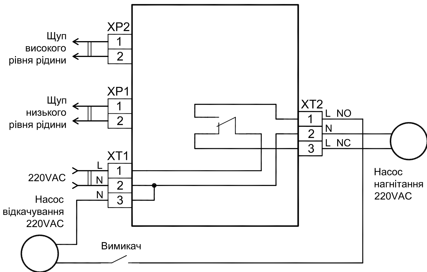
Схема підключення з двома насосами.
