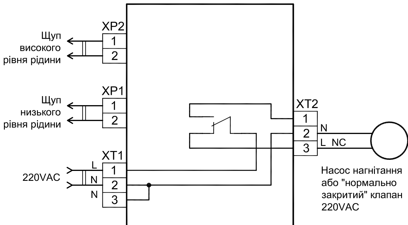
Схема підключення з одним насосом або запірним клапаном.
